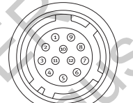
HIROSE HR10A-10R-12PB(71)
