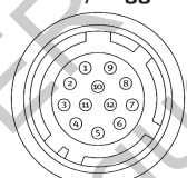
HIROSE HR10A-10R-12PB(71)
